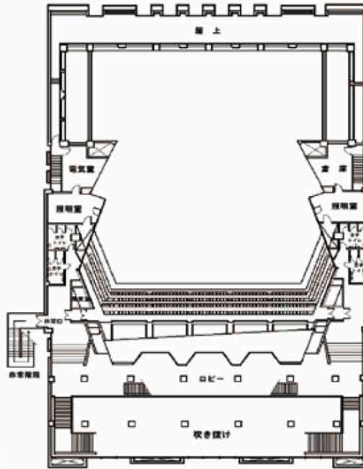
苫小牧市民会館 3階平面図
